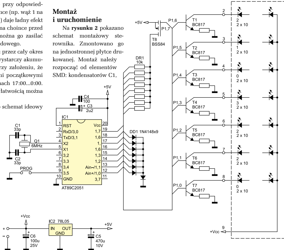
Rysunek 1. Schemat ideowy sterownika węży świetlnych
