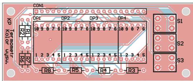
Rys. 3 Rozmieszczenie elementów na płytce drukowanej wyświetlaczy
